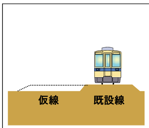
STEP1: 仮線用地を確保し、仮線を構築
