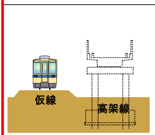
STEP3: 跡地に高架橋を構築
