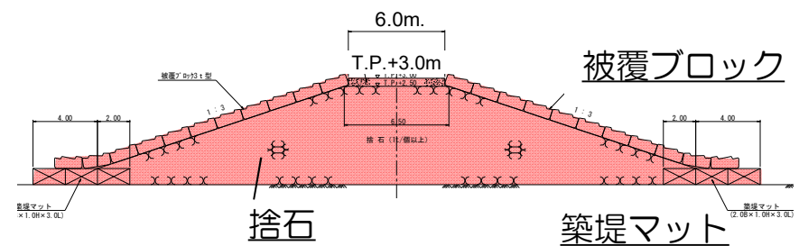
ヘッドランド 縦堤部 標準断面図
