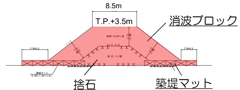
ヘッドランド 横堤部 標準断面図
